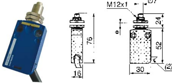
LL5XCMD21F0L1 (快动) LL5XCMD25F0L1 (慢动) M12 头金属形直动式
