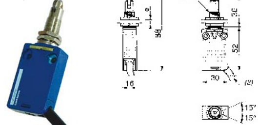
LL5XCMD2145L1 (快动) LL5XCMD2545L1 (慢动) 长度可调热塑滚轮摇杆
