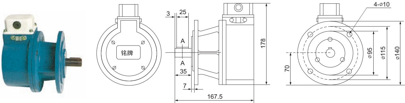
LLY1G-2T/□D型超速开关 LLY1G-2T/□D overspeed switch
