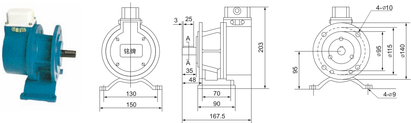
LLY1G-2T/□型超速开关 LLY1G-2T/□ overspeed switch
